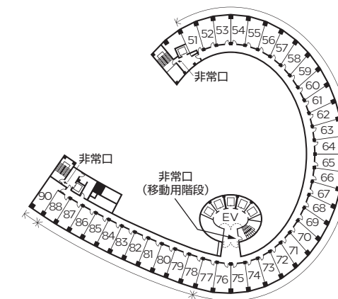
■ 客室階平面図（客室は基準階）
